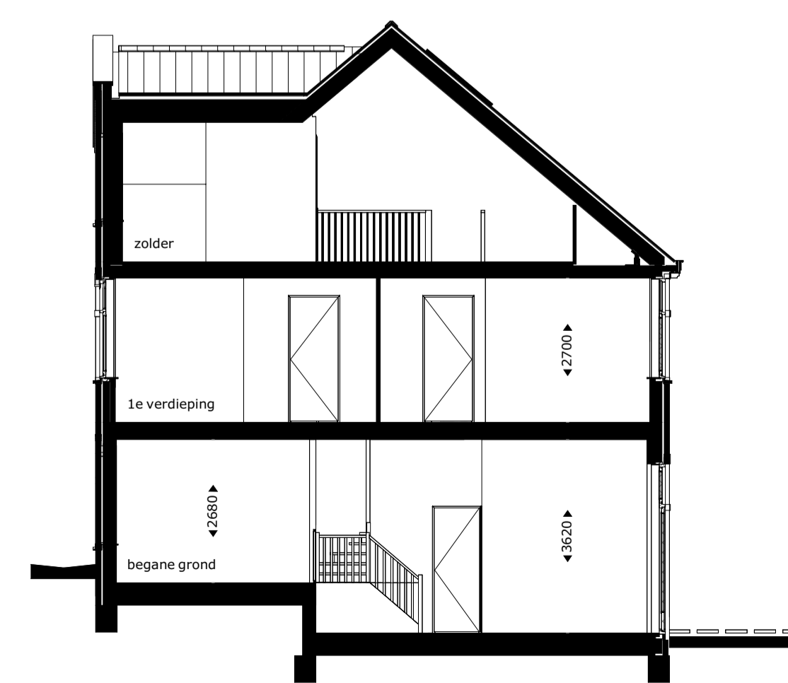
doorsnede A-A
