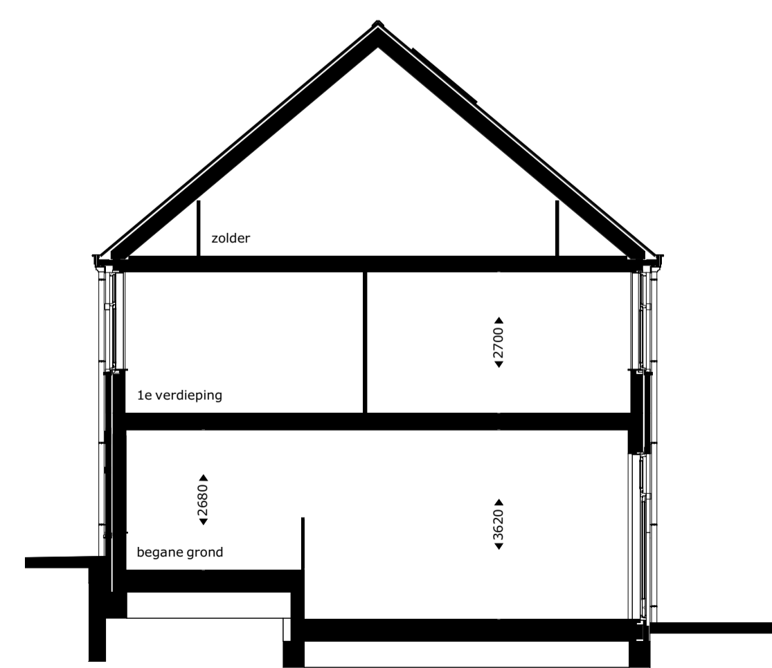
doorsnede B-B
