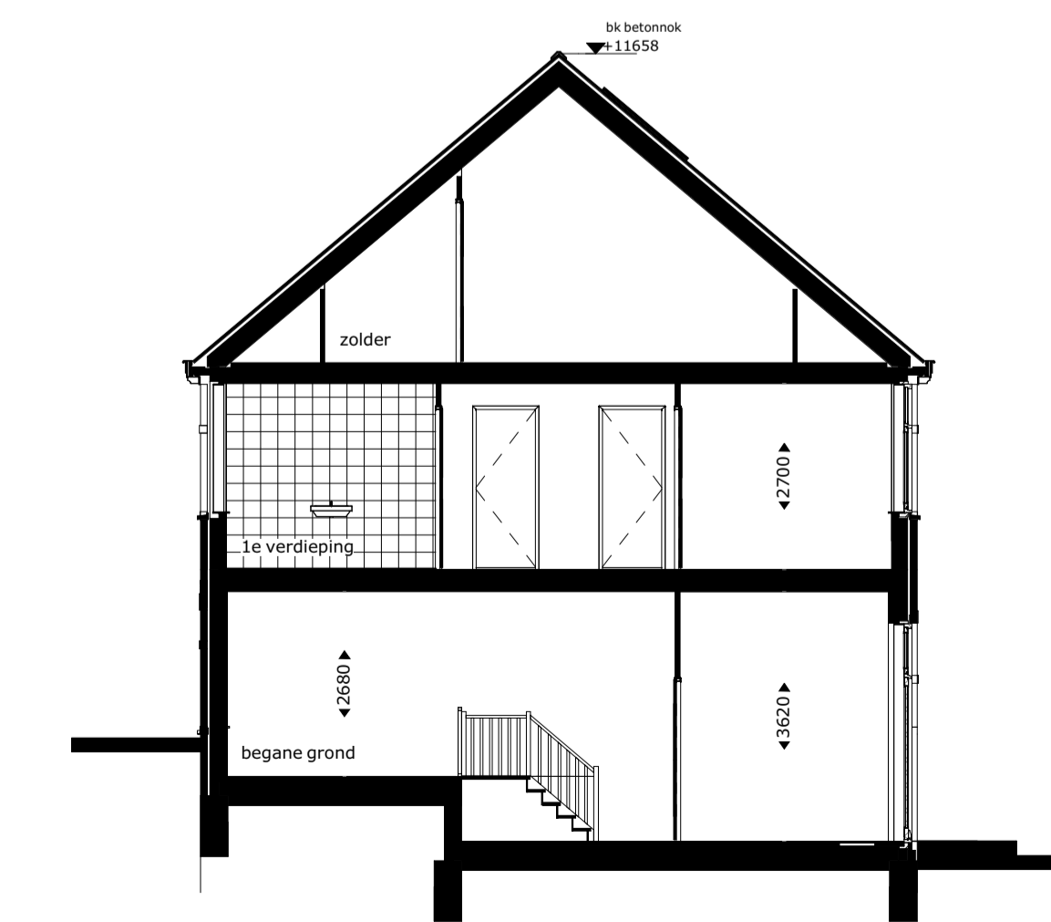
doorsnede D-D
