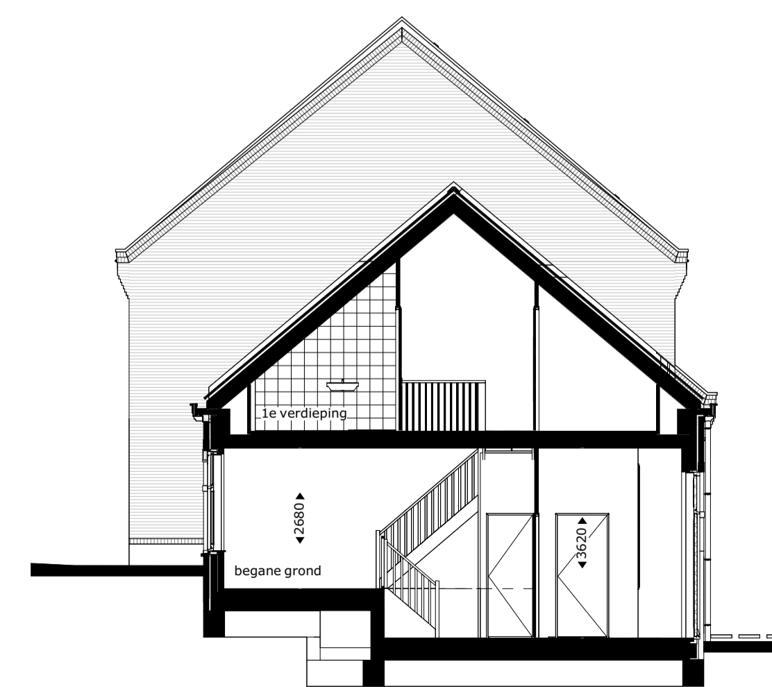
doorsnede C-C
