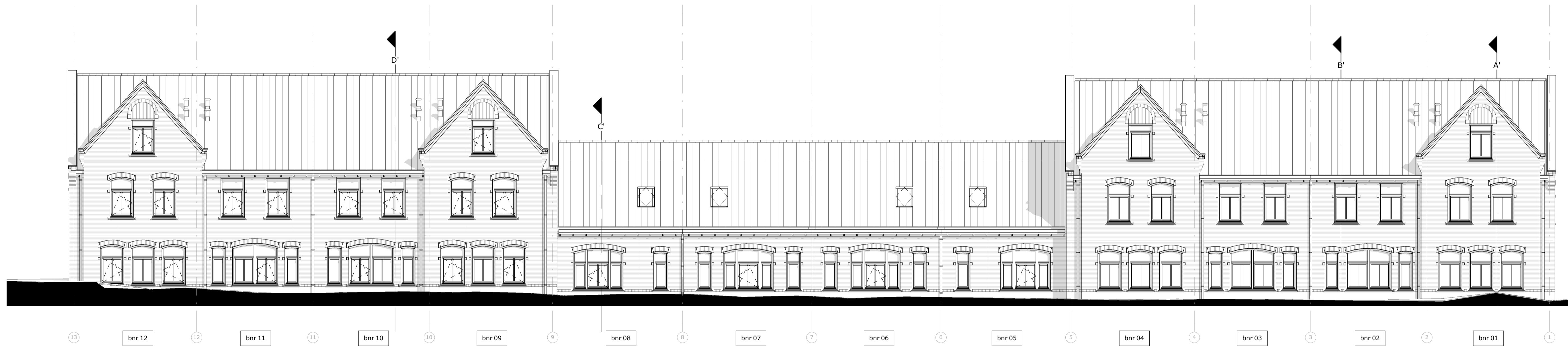
achtergevel
